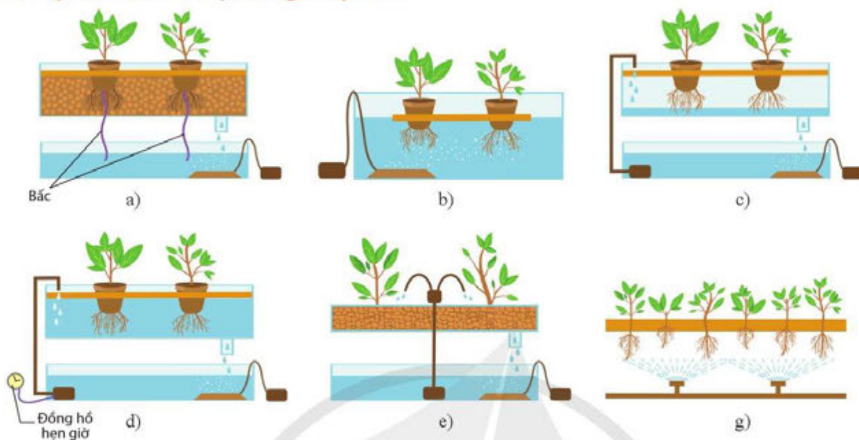
Hình 2.3. Một số mô hình hệ thống thủy canh phổ biến: hệ thống thủy canh dạng bậc (a), hệ thống thủy canh nước sâu (b), hệ thống thủy canh kỹ thuật màng mỏng dinh dưỡng (c), hệ thống thủy canh ngập và rút dinh kì (d), hệ thống thủy canh nhỏ giọt (e), hệ thống khí canh (g)
