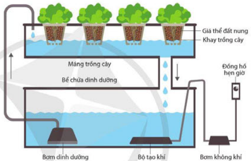
Hình 2.1. Hệ thống thủy canh
