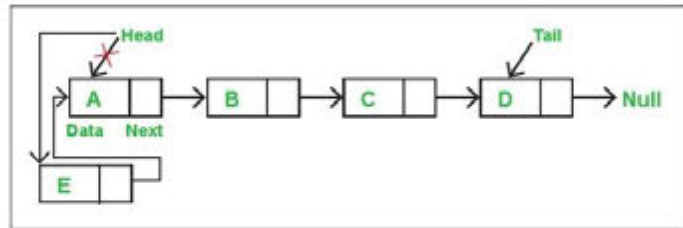
Hình 2a. Thêm nút vào đầu danh sách
