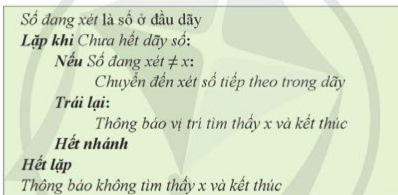
Hình 1. Thuật toán tìm kiếm tuần tự
